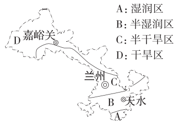
甘肃省干湿区分布
