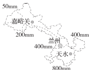
甘肃省年降水量分布
